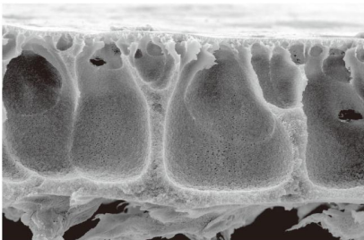
SUN®PVDF 平板膜片电镜图
